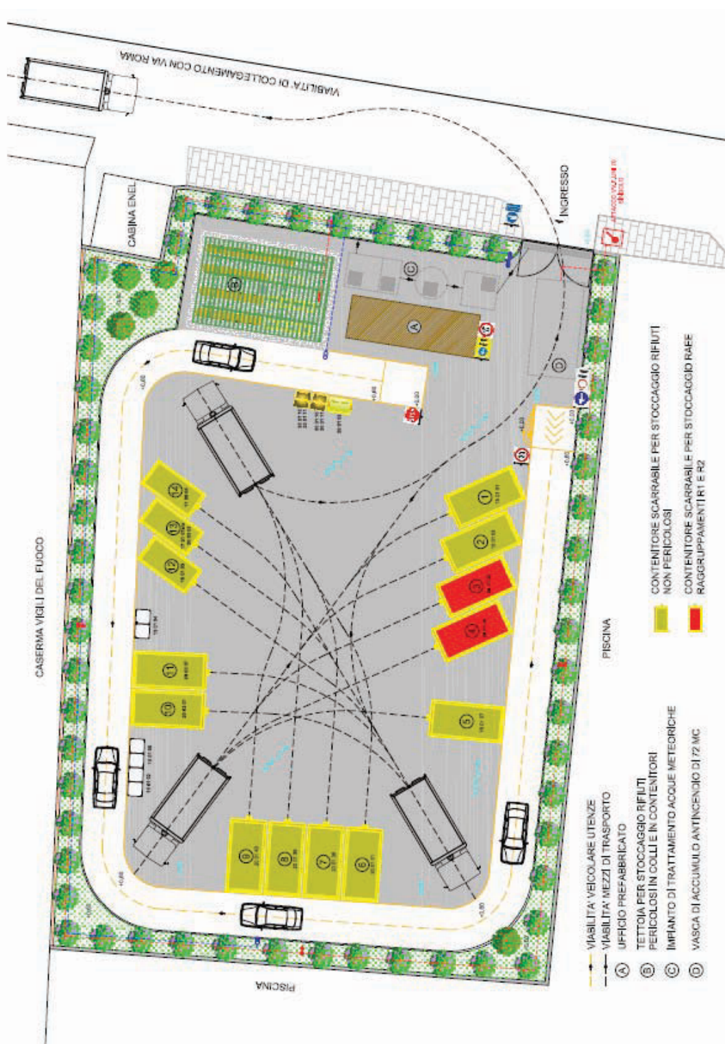
Figura 1 – Planimetria tipo di Centro Comunale di Raccolta
